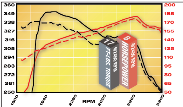
Dyno Chart: 1997 Ford F250 PSD
